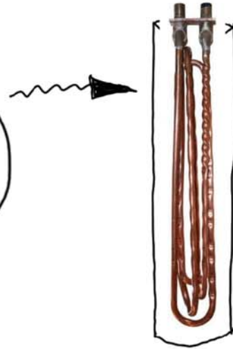
DRALLROHR
