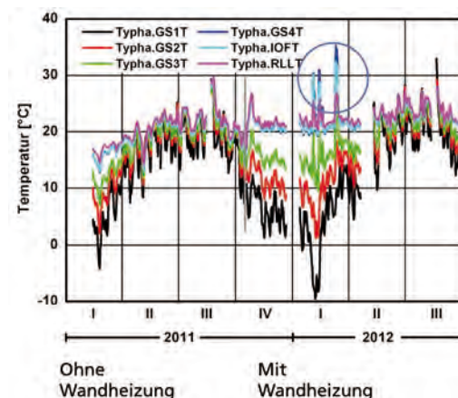
Bild 25: Gemessener Verlauf der Grenzschnitttemperaturen als Tagesmittelwerte für den Zeitraum von Januar 2011 bis September 2012, Diagramm IBP
