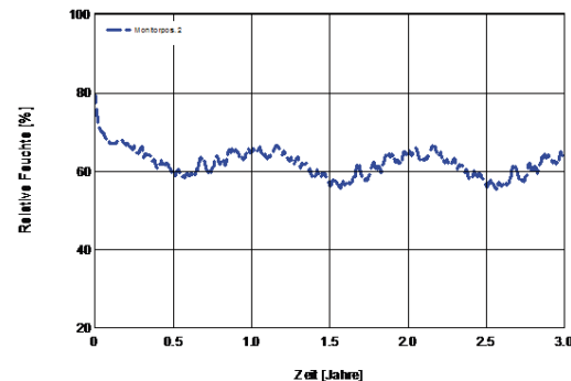
Bild 11: Zeitlicher Verlauf der Temperatur (links) und der relativen Luftfeuchte (rechts) zwischen Außenwand und Innendämmung, Diagramm IBP
