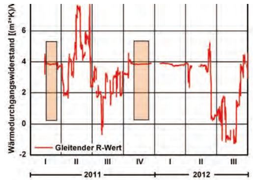
Bild 30: Aus den Messwerten (Bild 29) berechneter gleitender Wärmewiderstand (R-Wert). Die Balken zeigen Zeitbereiche, die für eine Beurteilung des Wärmewiderstandes geeignet sind, Diagramm IBP
