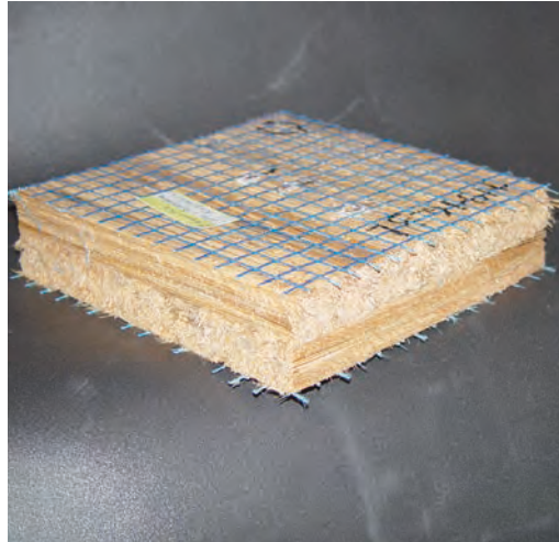
Bild 6: Plattenmaterial aus zwei senkrecht zueinander stehenden Schichten mit liegender Orientierung, zusammen mit den Materialkennwerten, Foto IBP
