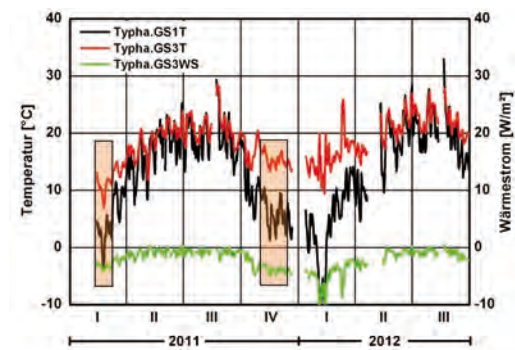
Bild 29: Hinter der Innendämmung (Grenzschicht 3) gemessener Wärmestrom zusammen mit dem Verlauf der Temperatur an der Grenzschicht 1 und 3. Die Balken zeigen Zeitbereiche, die für eine Beurteilung des Wärmewiderstandes geeignet sind, Diagramm IBP
