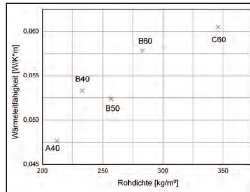
Bild 8: Wärmeleitfähigkeit der magnesitgebundenen Typhaplatte in Abhängigkeit von der Rohdichte, Diagramm IBP
