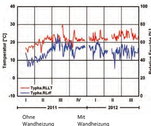
Bild 26: Gemessener Verlauf der Raumluftfeuchte und -temperatur, Diagramm IBP
