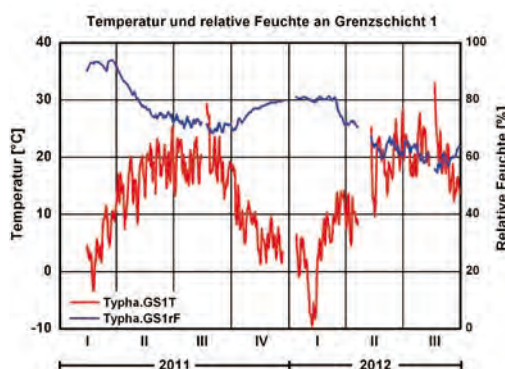
Bild 27: Verlauf der Temperatur und Feuchte an der Grenzschnitt 1, Diagramm IBP
