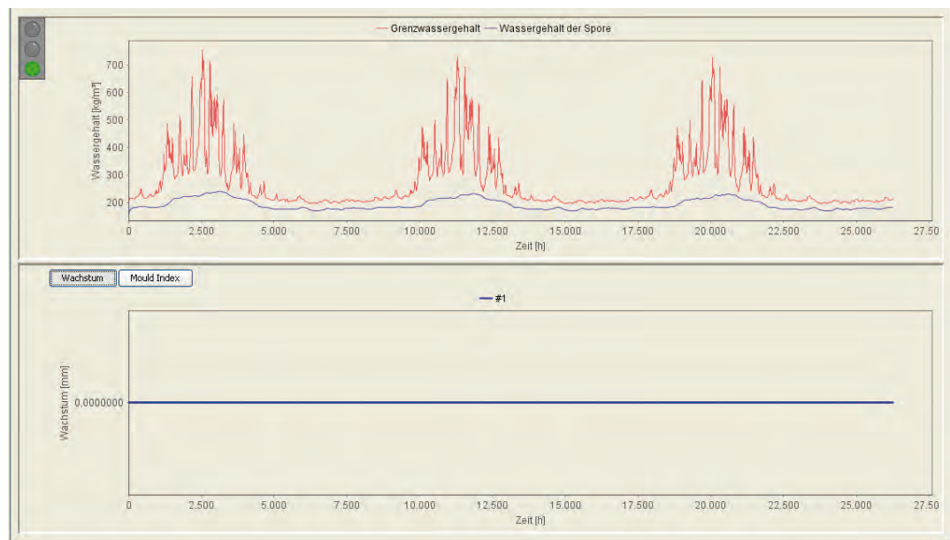
Bild 15: Ergebnis der Berechnungen mit WUFI®-Bio für den Bereich hinter der Innendämmung, Diagramm IBP
