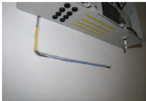
Bild 22: Unteransicht des Gerätekastens mit eingebautem Datenlogger (links) sowie der Unterseite mit Kombisensor für das Raumluftklima und Messausgängen für die Holzfeuchtemessungen und den in den Innenputz eingelassenen Sensor für die Innenoberflächentemperatur, Foto IBP
