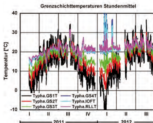
Bild 24: Verlauf der Grenzschnitttemperaturen als Stundenmittelwerte für den Zeitraum von Januar 2011 bis September 2012, Diagramm IBP
