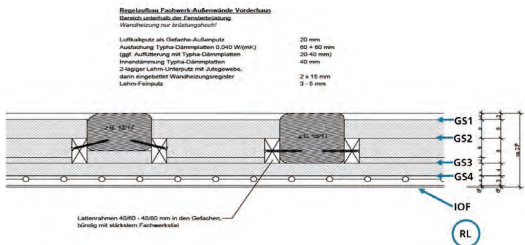
Bild 23: Schematischer Wandaufbau zusammen mit der Position der Grenzschichten bzw. Messstellen, Plangrundlage Architekturbüro Fritsch+KnodtKlug
