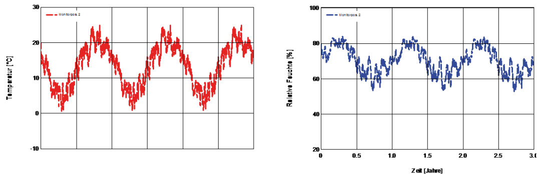
Bild 14: Zeitlicher Verlauf der Temperatur (oben) und der relativen Luftfeuchte (unten) zwischen Außenwand und Innendämmung bei einer Hinterströmung mit 1 m³/md, Diagramm IBP
