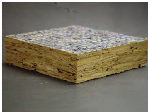
Bild 5: Chip-Board mit überwiegend waagrecht zur Plattenebene orientierten, gröberen Partikel, zusammen mit den Materialkennwerten, Foto IBP
