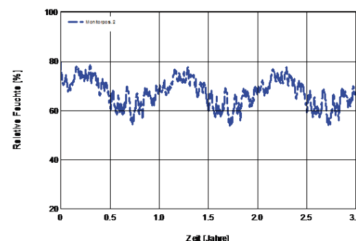
Bild 13: Zeitlicher Verlauf der Temperatur (links) und der relativen Luftfeuchte (rechts) zwischen Außenwand und Innendämmung bei einer Hinterströmung mit 1 l/mh, Diagramm IBP
