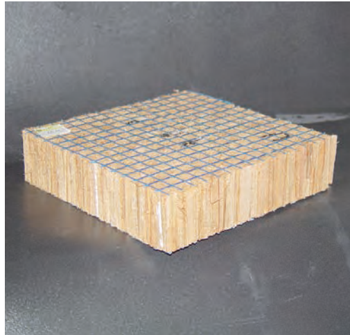
Bild 3: Plattenmaterial mit senkrecht zur Plattenebene orientierten stabförmig aus der Blattmasse geschnittener Partikel, zusammen mit den Materialkennwerten, Foto IBP
