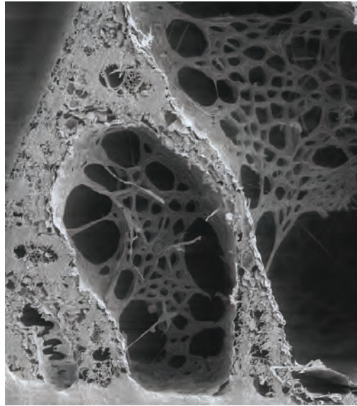
Unterschiedliche Kammerdimensionen und Ausformungen von vertikalen Stützwänden, Aufnahme: Chr. Gruber, BLfD Zentrallabor
