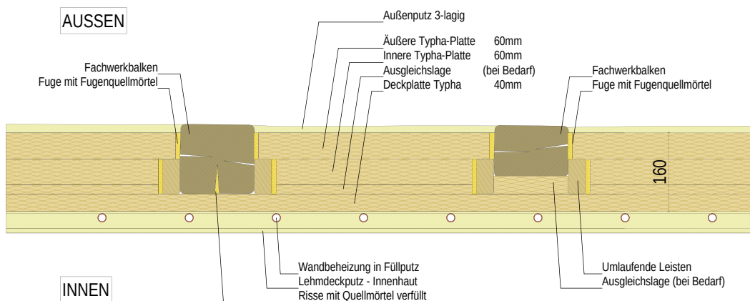
Mitte: Grundriss Wandaufbau, Plangrundlage Architekturbüro Fritsch+Knodt&Klug
