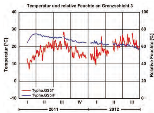
Bild 28: Verlauf der Temperatur und Feuchte an der Grenzschicht 3, Diagramm IBP
