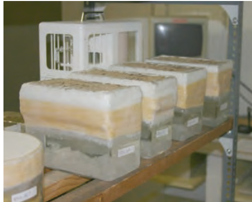
Bild 2: Auf die Prüfgefäße dicht aufgebrachte Typha-Platten während der Diffusionswiderstandsmessung, Foto IBP
