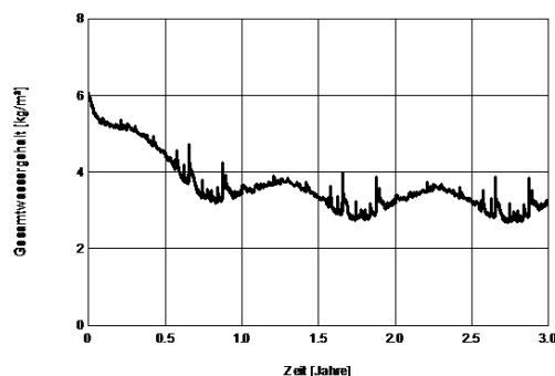
Bild 10: Berechneter Verlauf des Gesamtwassergehaltes der innenseitig mit der Typhaplatte gedämmten Außenwand, Diagramm IBP.
